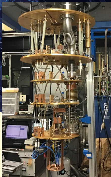
量子コンピュータ研究設備
